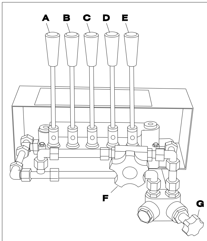
56 HYDRAULISCHE BEDIENINGSORGANEN
