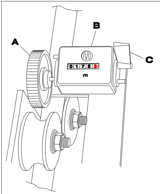
23 METERTELLER
