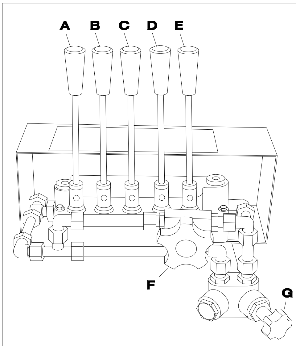
56 HYDRAULISCHE BEDIENINGSORGANEN
