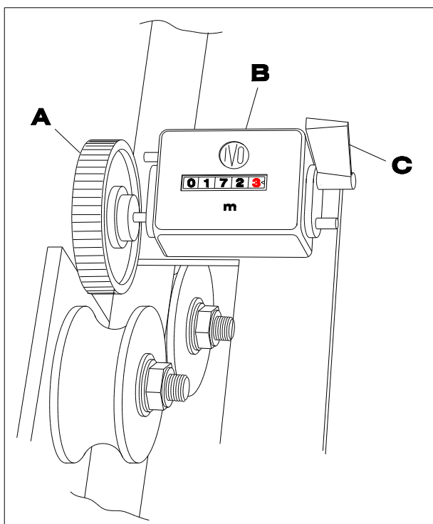
23 METERTELLER
