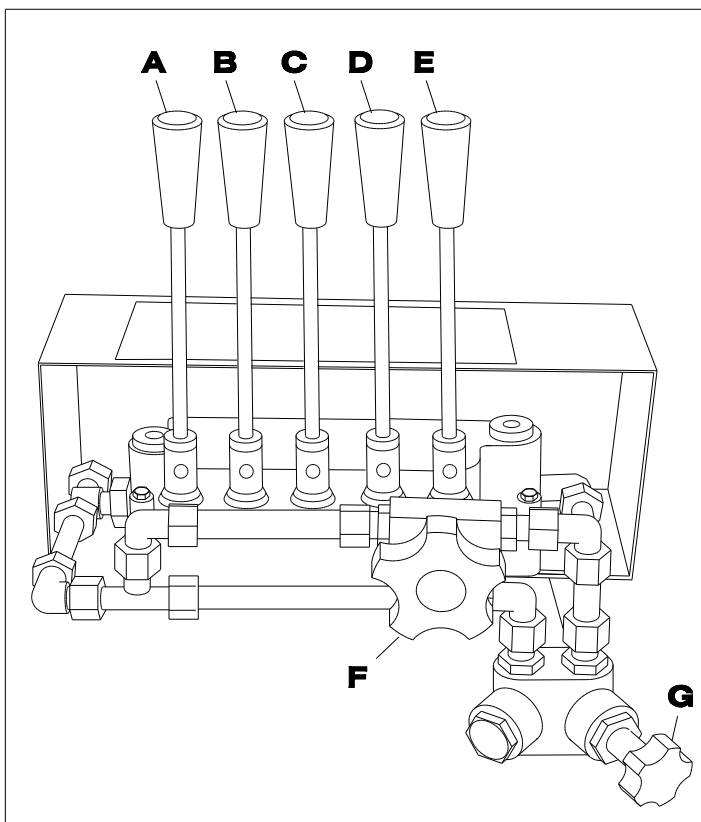
56 HYDRAULISCHE BEDIENINGSORGANEN
