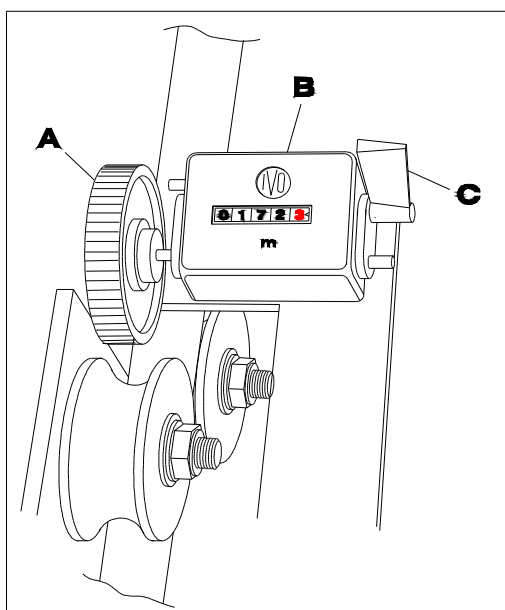
53 METERTELLER
