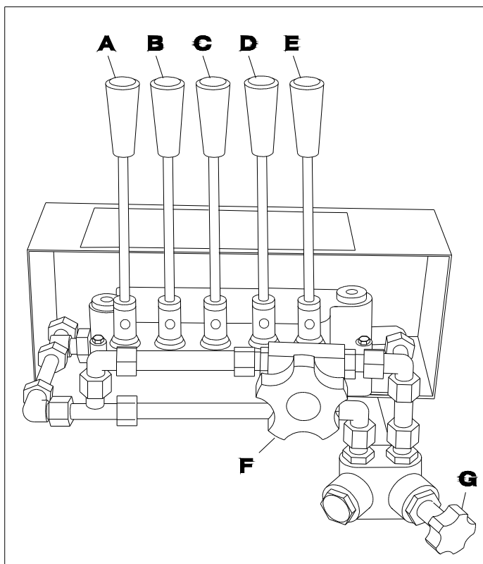
56 HYDRAULISCHE BETRIEBSORGANE
