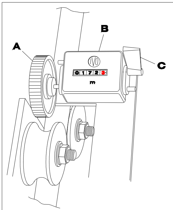
23 METERTELLER
