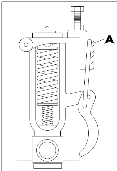
05 SPOELWATERDRUK REGELAAR
