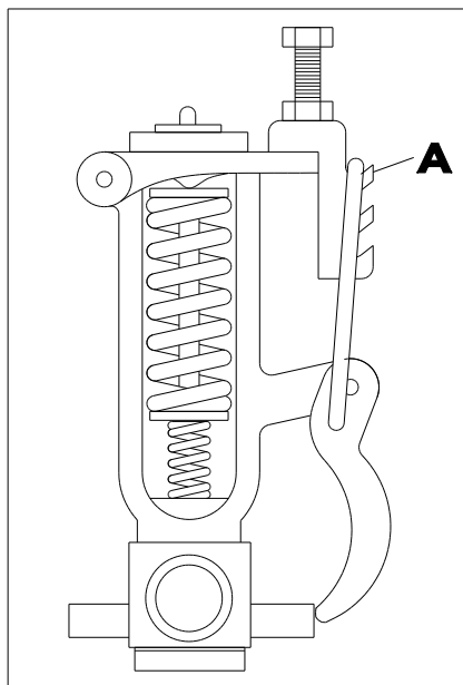
05 SPOELWATERDRUK REGELAAR
