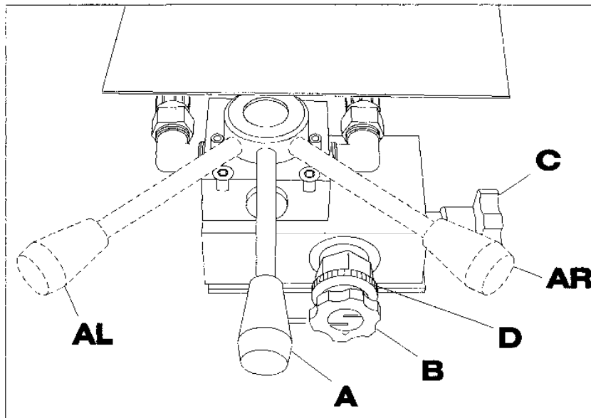
38 HYDRAULISCHE BETRIENINGS-ORGANEN
