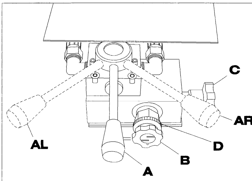
38 HYDRAULISCHE BEDIENTINGS-ORGANEN
