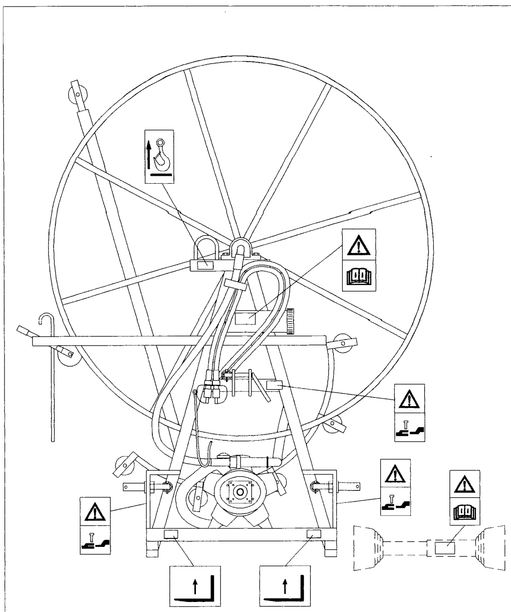
33 LOCATIE STICKERS VOORZIJDE
