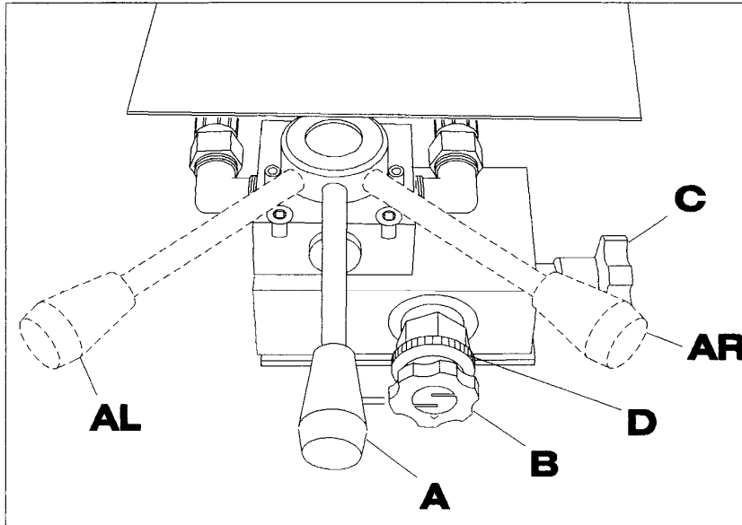
38 HYDRAULISCHE BEDIENINGS-ORGANEN
