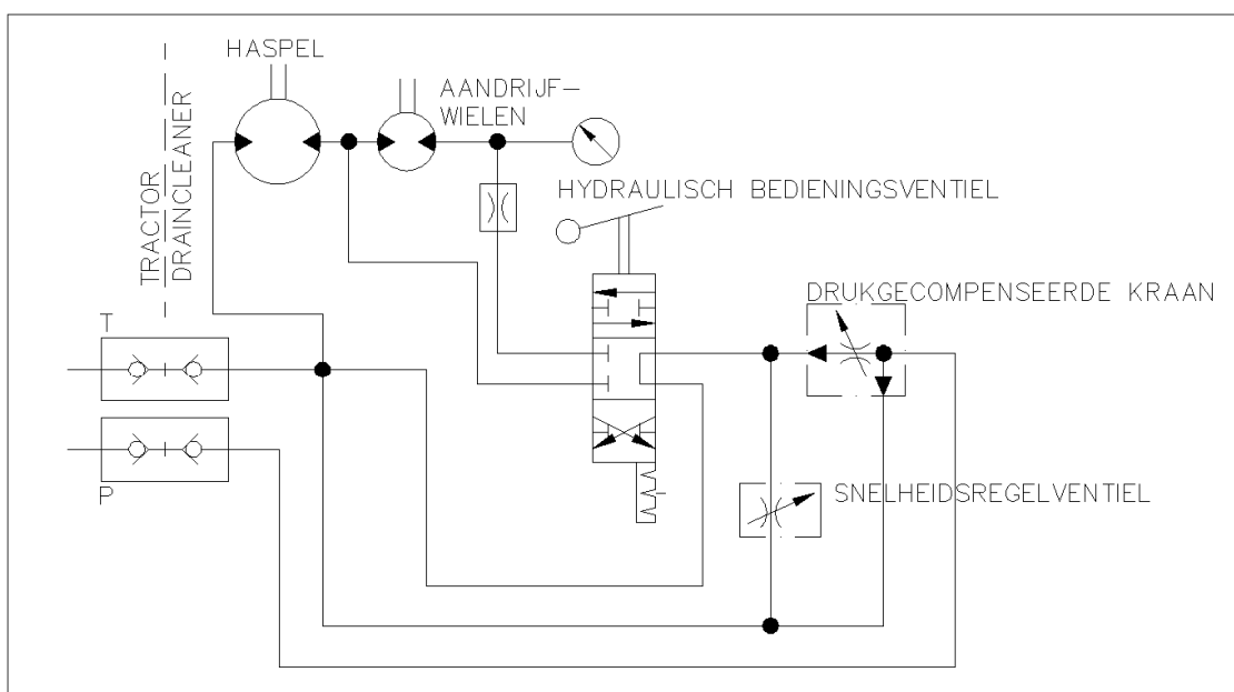
28 HYDRAULISCH SCHEMA JUNIOR
