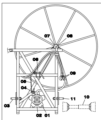
20 HOOFDCOMPONENTEN VOORZIJDE DELTA
