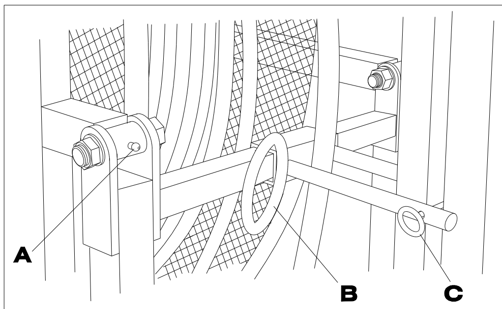
22 ARMBORGSTEUN/SPOELSLANGGELEIDER
