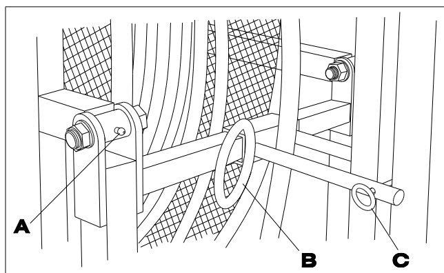
22 ARMBORGSTEUN/SPOELSLANGELEIDER
