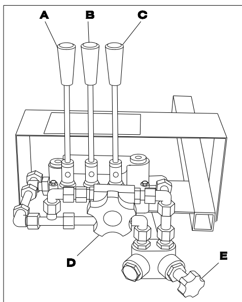
21 HYDRAULISCHE BEDIENINGSORGANEN
