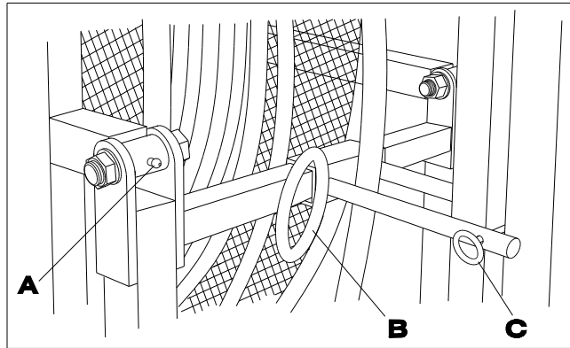
22 ARMBORGSTEUN/SPOELSLANGELEIDER
