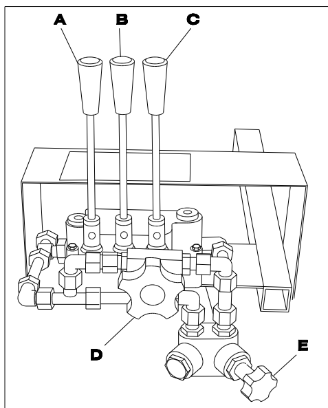
21 HYDRAULISCHE BEDIENUNGSORGANEN
