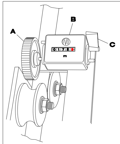
23 METERTELLER
