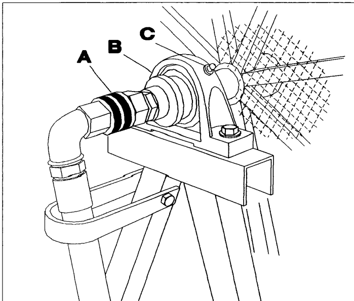
41 HASPELLAGER EN WATERKOPPELING
