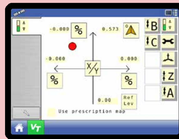
▲ SmartLEVEL instellingenpagina
